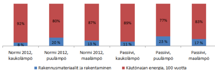
Energian ja rakentamisen osuus elinkaaren hiilijalanjäljessä
